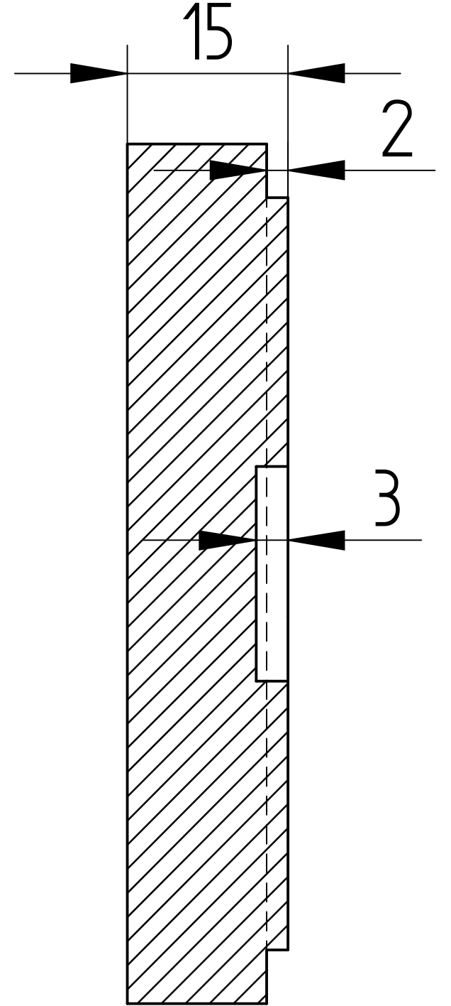
SECTION A-A
